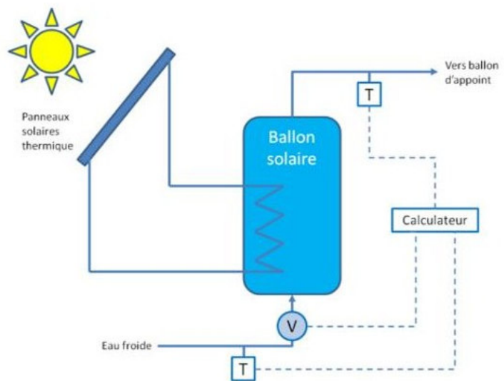
Schéma simplifié d'un suivi d'installation solaire thermique
